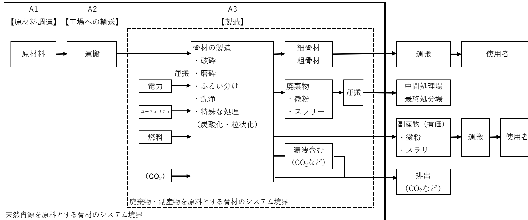
付録図 A-1 骨材のライフサイクルフローおよびシステム境界図
